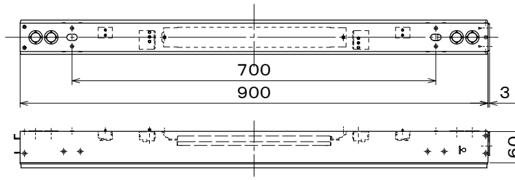
全体図
